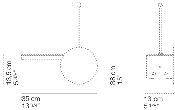
Fischietto R
